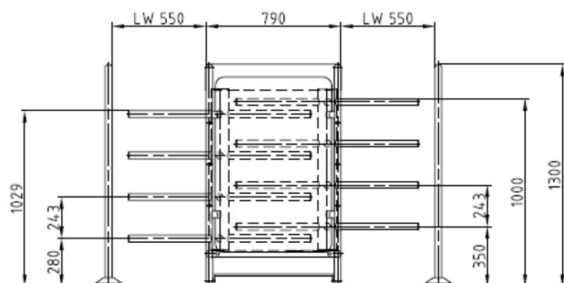
Lane dividers optional
