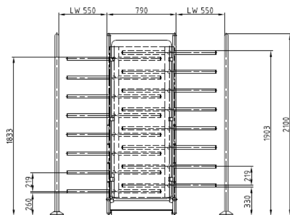
Spurteiler optional
